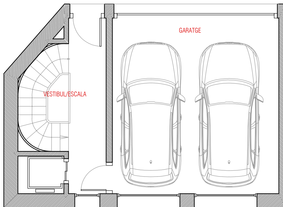
PLANTA SEGONA
