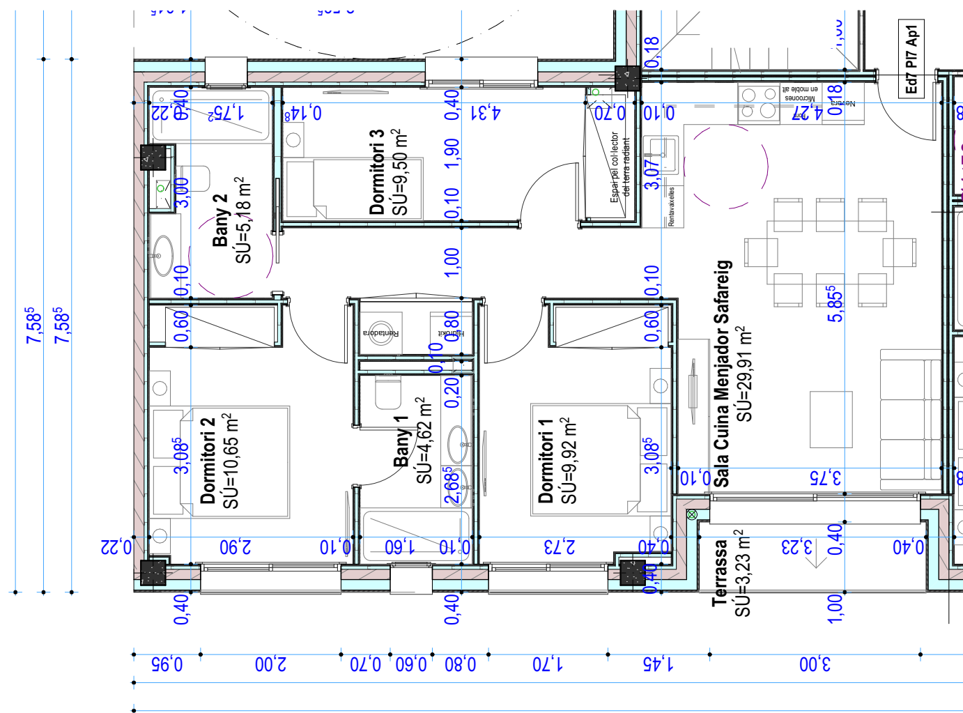
Ed7 PI07 Ap1 (s/Terr.) SC=83,72 m²
