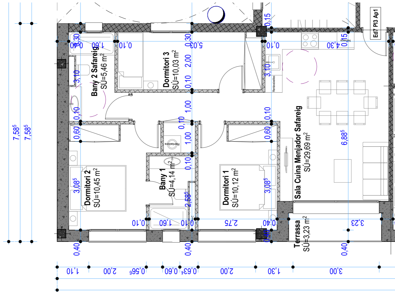
Ed7 PI03 Ap1 (s/Terr.) SC=83,67 m 2
