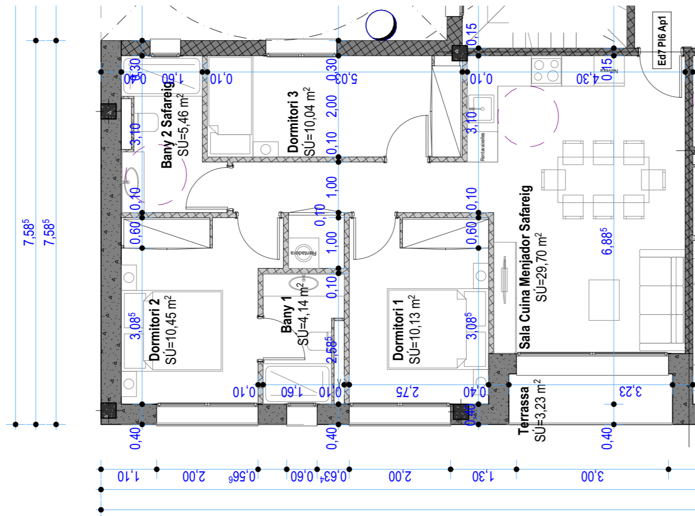
Ed7 PI06 Ap1 (s/Terr.) SC=83,67 m 2
