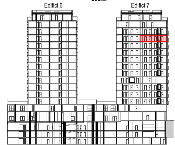
Secció
